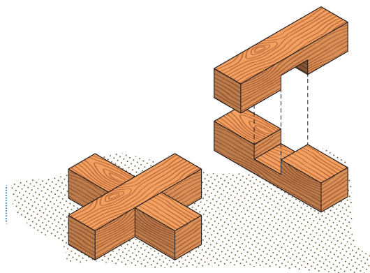
COUPE MI-BOIS
