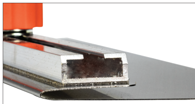
Le bord replié forme un arrondi aidant la mise en place d'une fibre : idéal pour doser la pression et ainsi lisser l'enduit sans trace de reprise.
